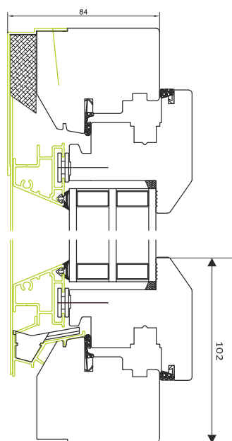
Övre/nedre karm
