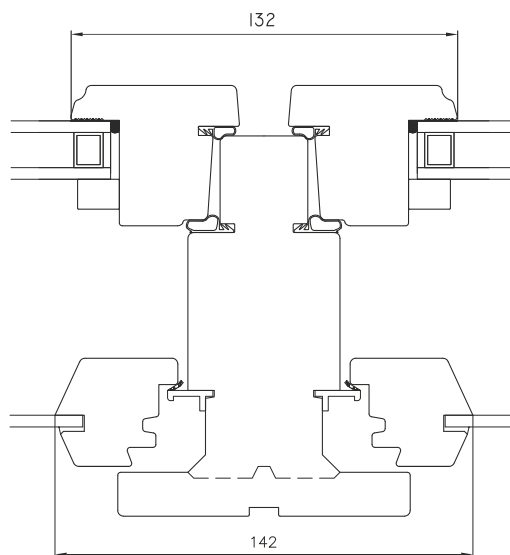
Vertikal impost
